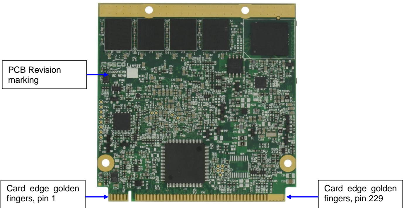
Bottom side
