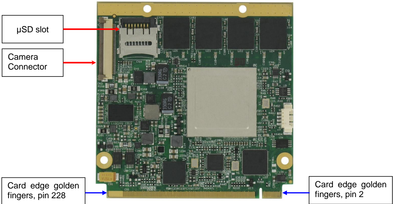
Bottom side
