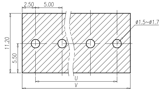
P.C.B. LAYOUT (S=4:1)
