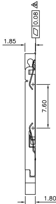
△ Section A-A
